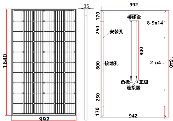
组件尺寸
