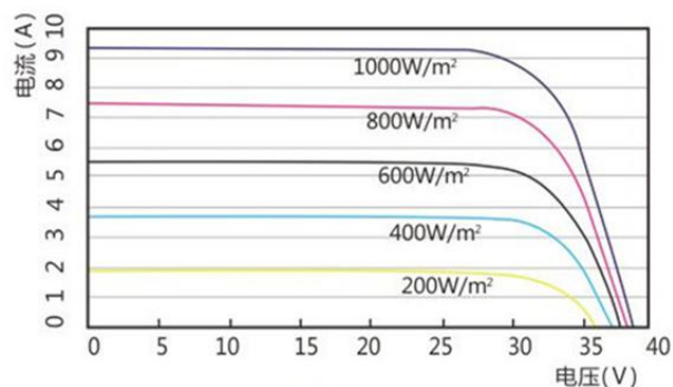
I-V 曲线
